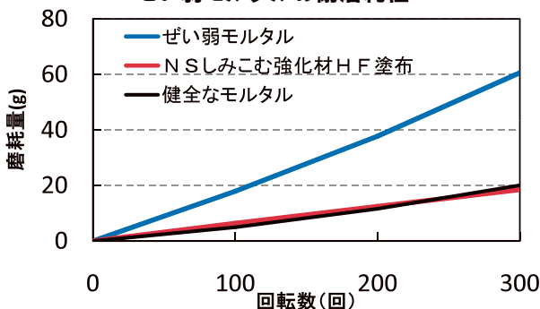
ぜい弱モルタルの耐磨耗性
